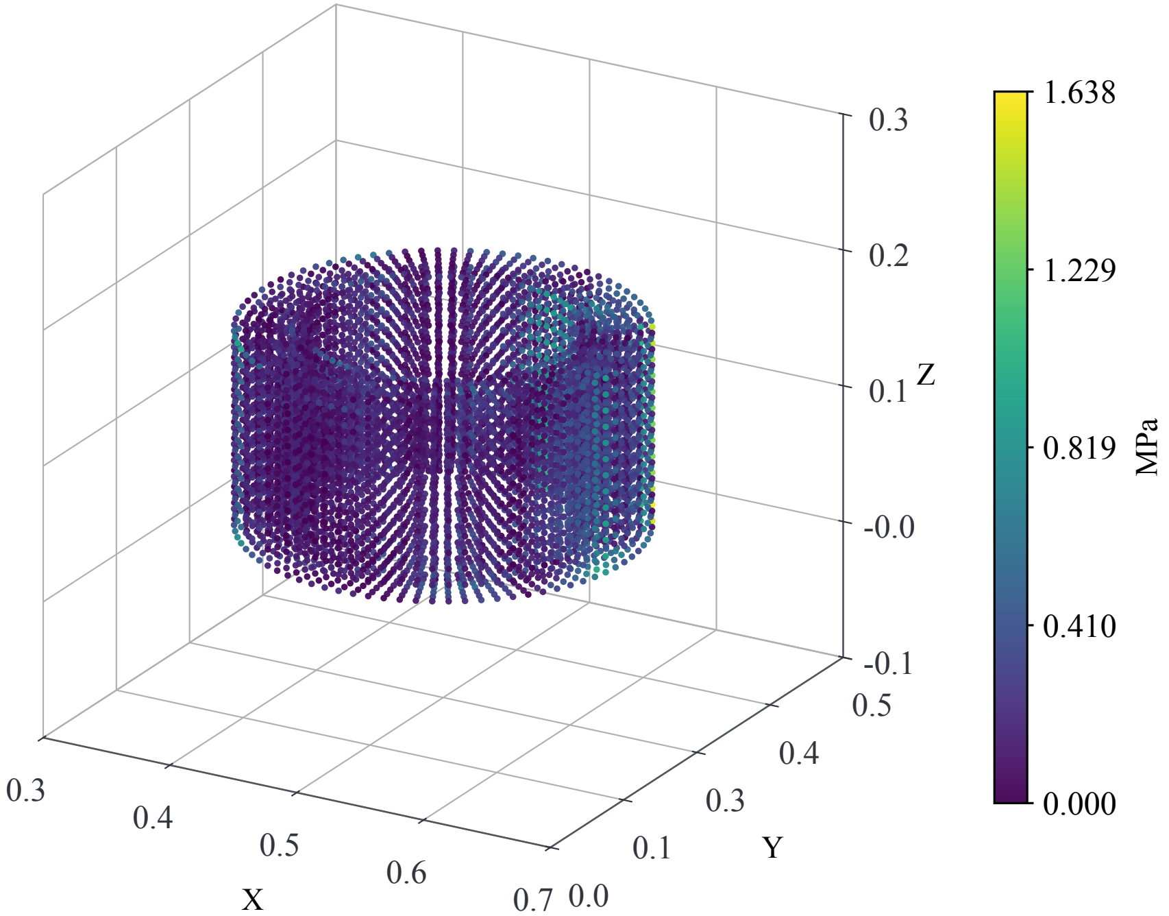
Absolute Error
